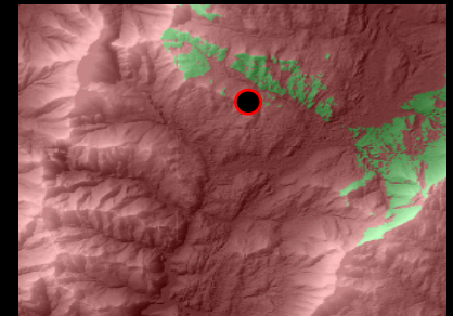
Visibilité / Inter-visibilité
